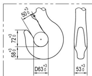
Hook dimensions DIN15401-2.5T
