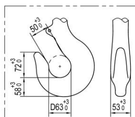
Hook dimensions DIN15401-2.5T
