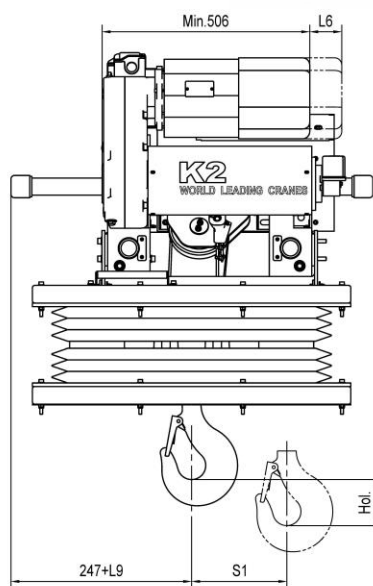
Hook dimensions DIN15401-5V
