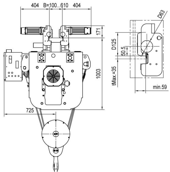
Hook dimensions DIN15401-5V
